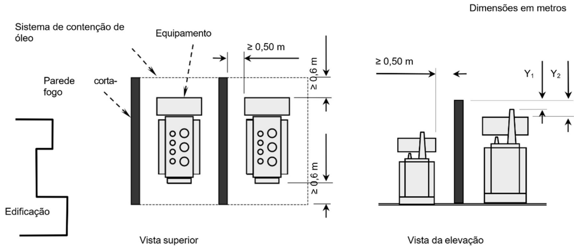
Figura A.5: Separação por parede tipo corta-fogo entre equipamentos e edificação
