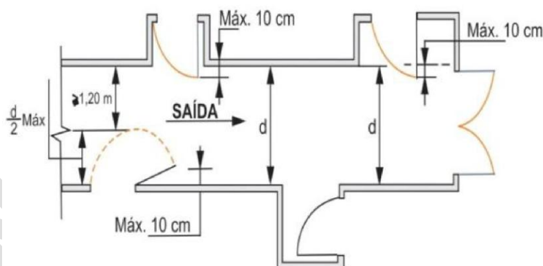
Figura 2: Abertura das portas no sentido de saída
