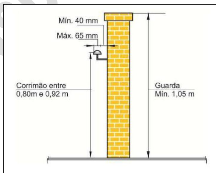
Figura 22: Dimensões de guardas e corrimãos
