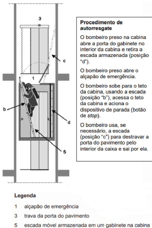
Figura 25: Desenho esquemático do alçapão
