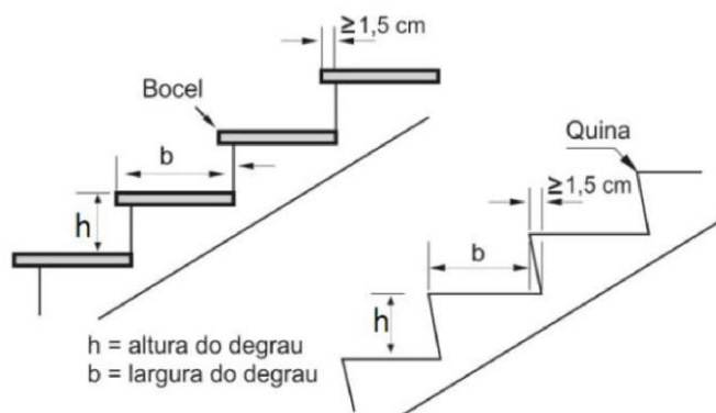
Figura 4: Altura e largura dos degraus
