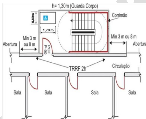
Figura 20: Escada aberta externa
