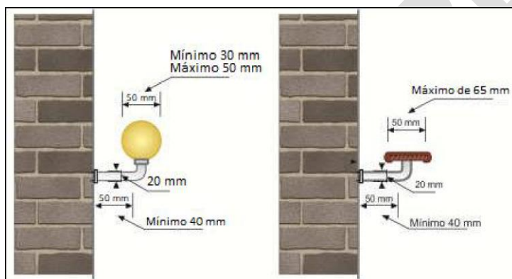
Figura 23: Pormenores de corrimãos
