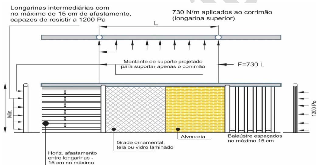
Figura 24: Pormenores construtivos da instalação de guardas e as cargas a que elas devem resistir
