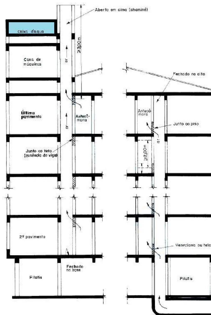
Figura 18: Exemplo de dutos de ventilação (corte AB e corte CD)
