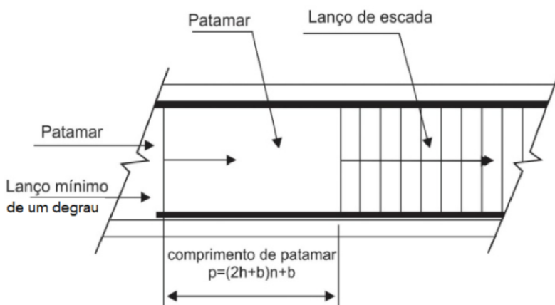
Figura 5: Lanço mínimo e comprimento de patamar
