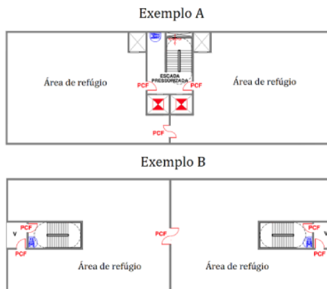
Figura 29: Desenho esquemático da área de refúgio
