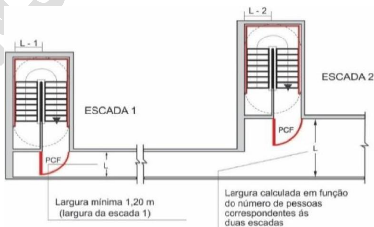
Figura 30: Dimensionamento de corredores de descarga
