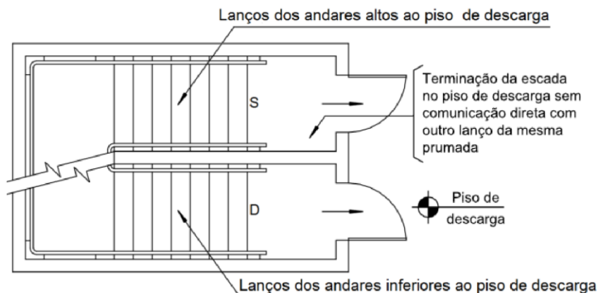
Figura 3: Segmentação das escadas no piso da descarga
