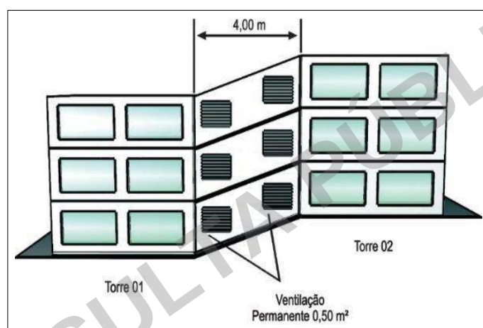
Figura 13: Abertura lateral na escada
