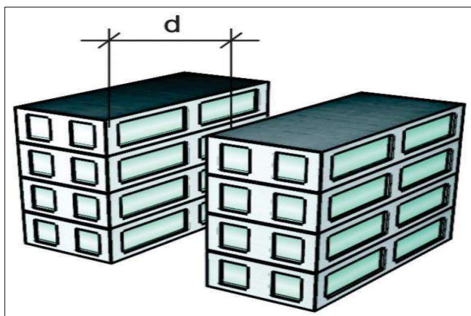
Figura 6: Distância de segurança
