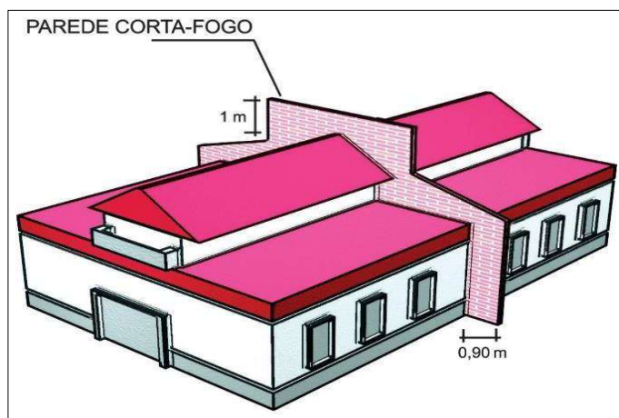
Figura 8: Parede corta-fogo
